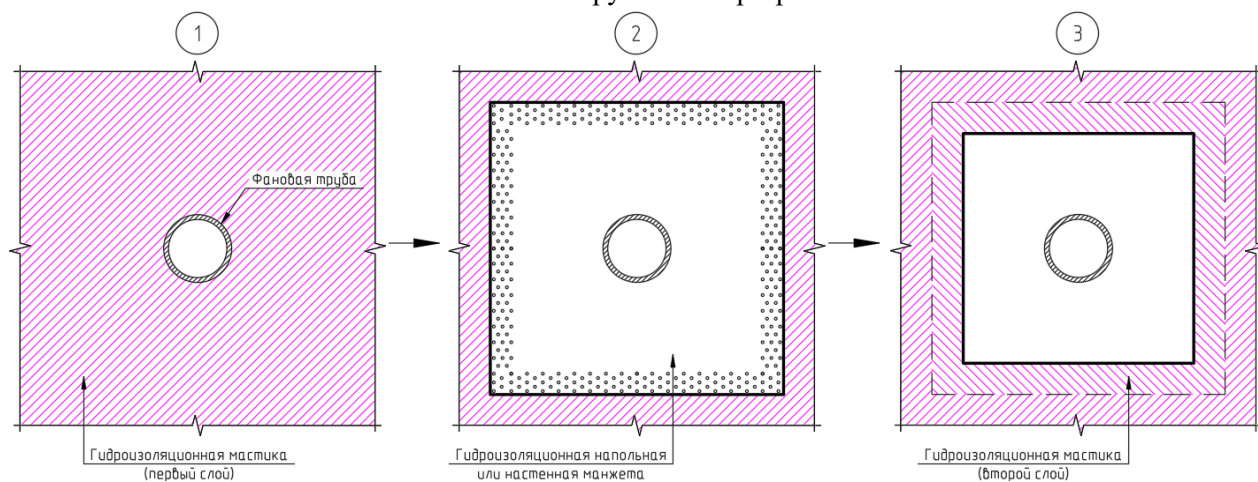
Рис.14.4. Последовательность нанесения гидроизоляционной манжеты.
