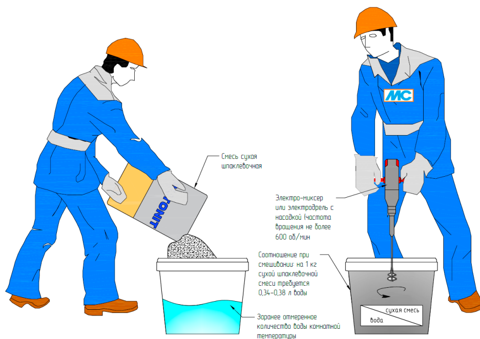
Рис. 16. Организация работ по затворению сухой шпаклевочной смеси
