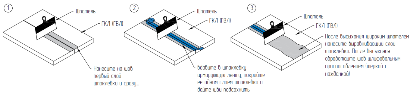
Рис. 18. Порядок шпаклевки швов между листов ГКЛ (ГВЛ) с использованием армирующей сетки
