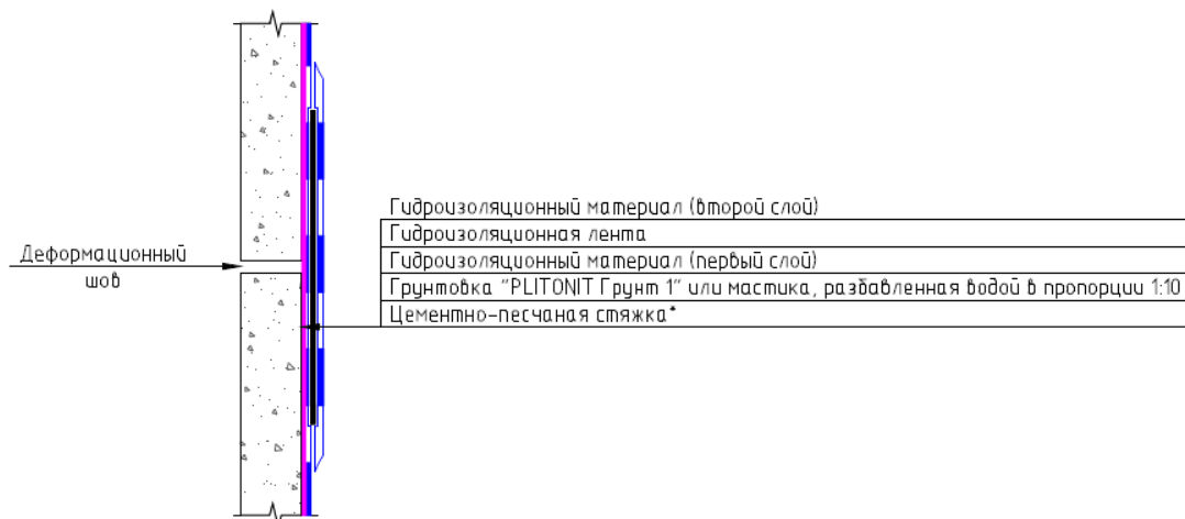
Рис.14.3. Конструктивный разрез №3.
