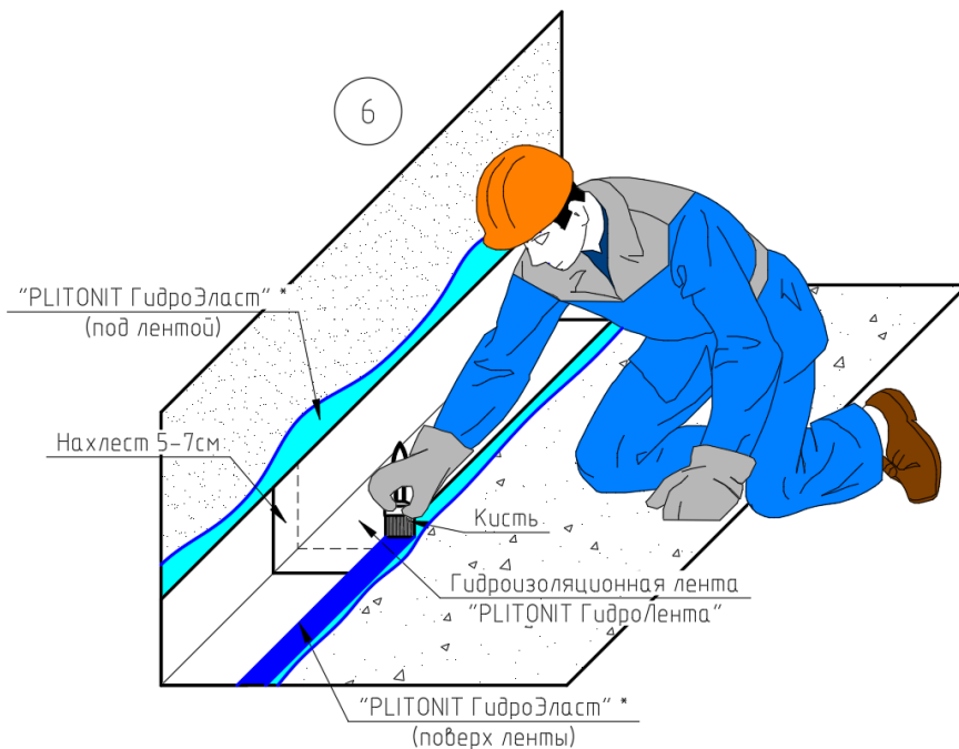
Рис.15.1. Последовательность работ (на стенах работа в аналогичном порядке), где: 1 - проверка ровности основания контрольной рейкой (аналогично для горизонтальной поверхности); 2 – размешивание емкости с мастикой; 3 – нанесение первого слоя мастики, разбавленной водой в пропорции 1:10, на основание; 4 – нанесение гидроизоляции на поверхность (аналогично для горизонтальной поверхности); 5 – укладка гидроизоляционной ленты на поверхность, предварительно обработанную «PLITONIT ГидроЭласт» или «PLITONIT WaterProof Standard»; 6 – поверхностная обработка ленты мастикой «PLITONIT ГидроЭласт» или «PLITONIT WaterProof Standard».
